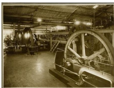
Gambar 2. Mesin Pengolahan Gula di Pabrik Meritjan (Sumber: digitalcollections.universiteitleiden.nl )
