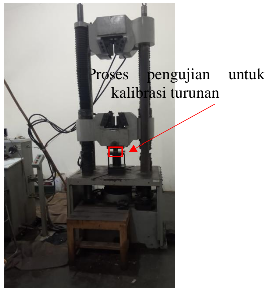
Gambar 15. Proses pengujian bahan uji untuk kalibrasi turunan pada mesin Universal Testing machine (UTM)
