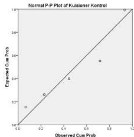
Gambar 1. P-P plot dan Q-Q plot Data Kuisioner Kelompok Kontrol
