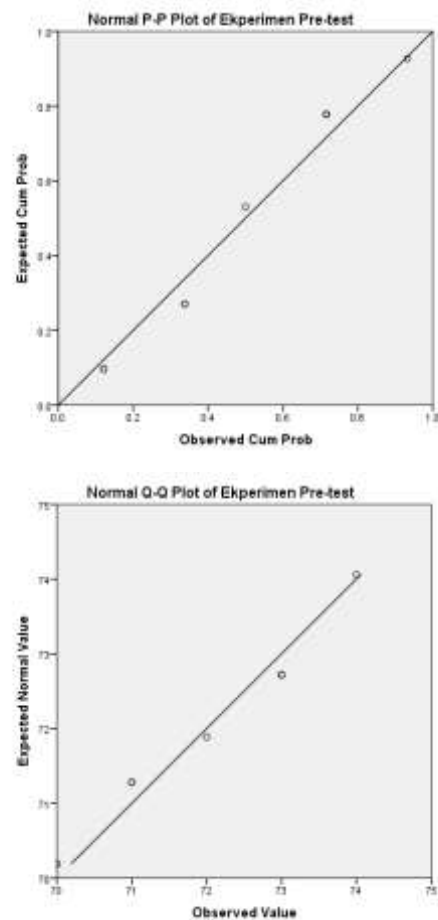
Gambar 4. P-P plot dan Q-Q plot Data Pretest Kelompok Eksperimen
