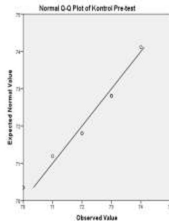
Gambar 3. P-P plot dan Q-Q plot Data Pretest Kelompok Kontrol
