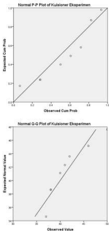
Gambar 2. P-P plot dan Q-Q plot Data Kuisioner Kelompok Eksperimen
