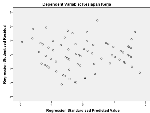
Gambar 3. Uji heterokedastisitas
